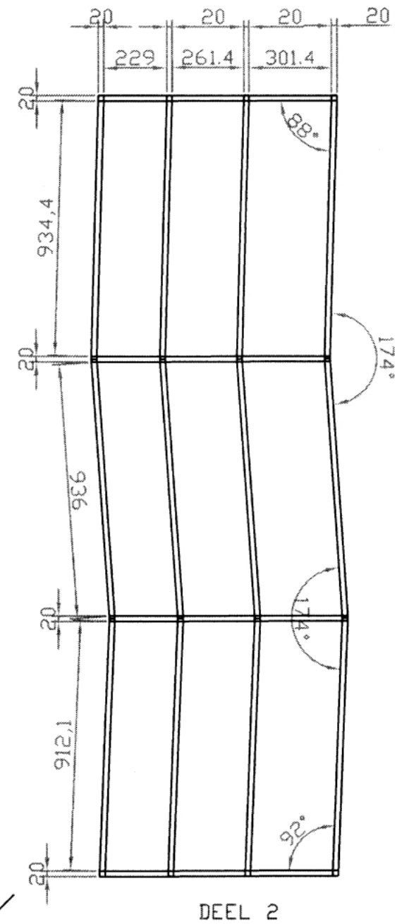
SCHAAL 1:30
