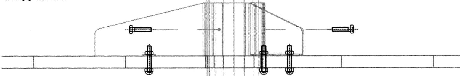
bevestiging tussenblad 1:2
