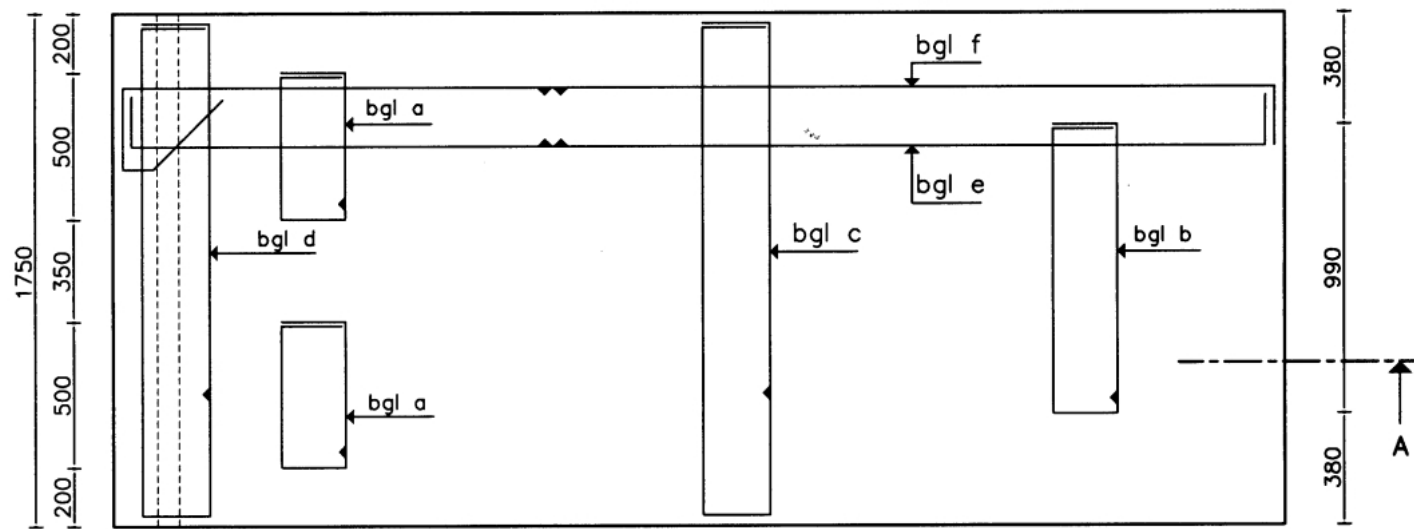
BOVENAANZICHT
