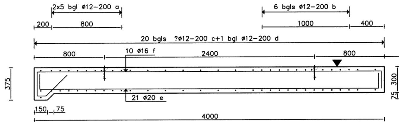
ZIJAANZICHT
