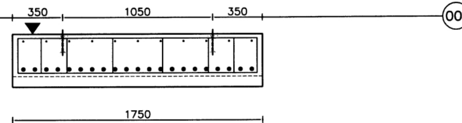
DOORSNEDE
