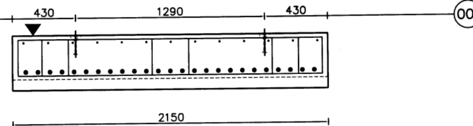
DOORSNEDE
