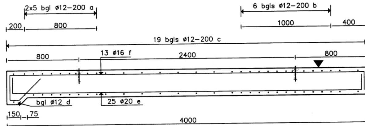
ZIJEAANZICHT
