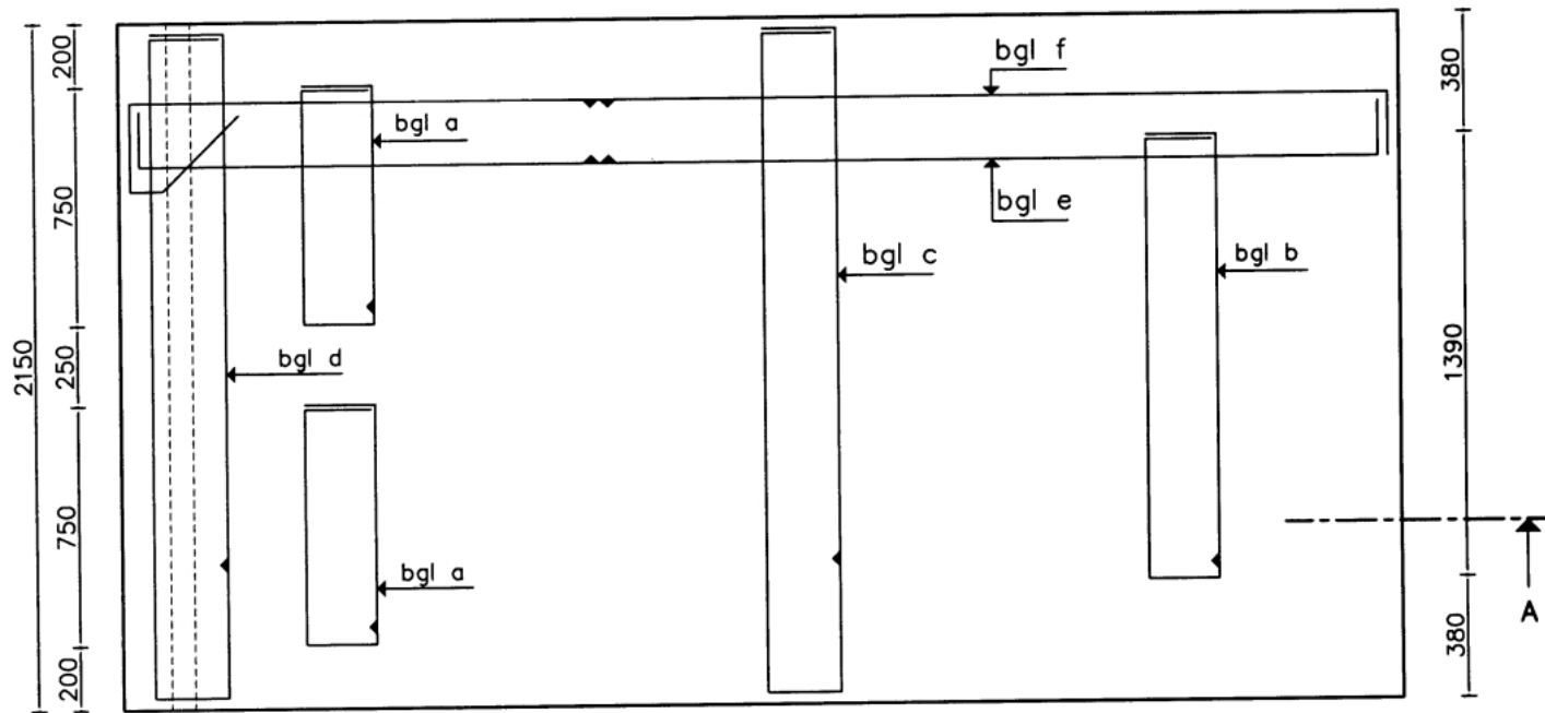
BOVENAANZICHT
